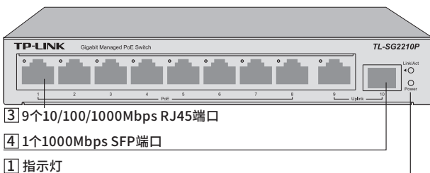
图1-6 TL-SG2210P前面板示意图
