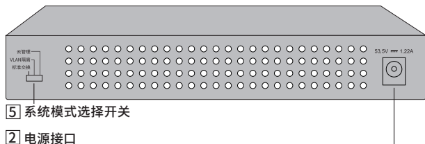
图1-7 TL-SG2210P后面板示意图
